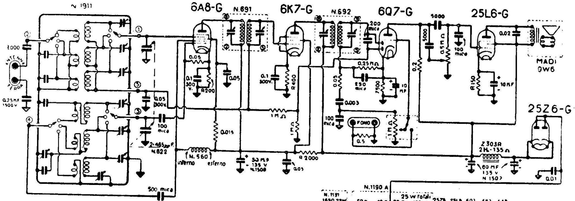
RICEVITORE SUPER G.53 ONDE CORTE - MEDIE - LUNGHE 110 - 220 VOLT C.C. - C.A.
